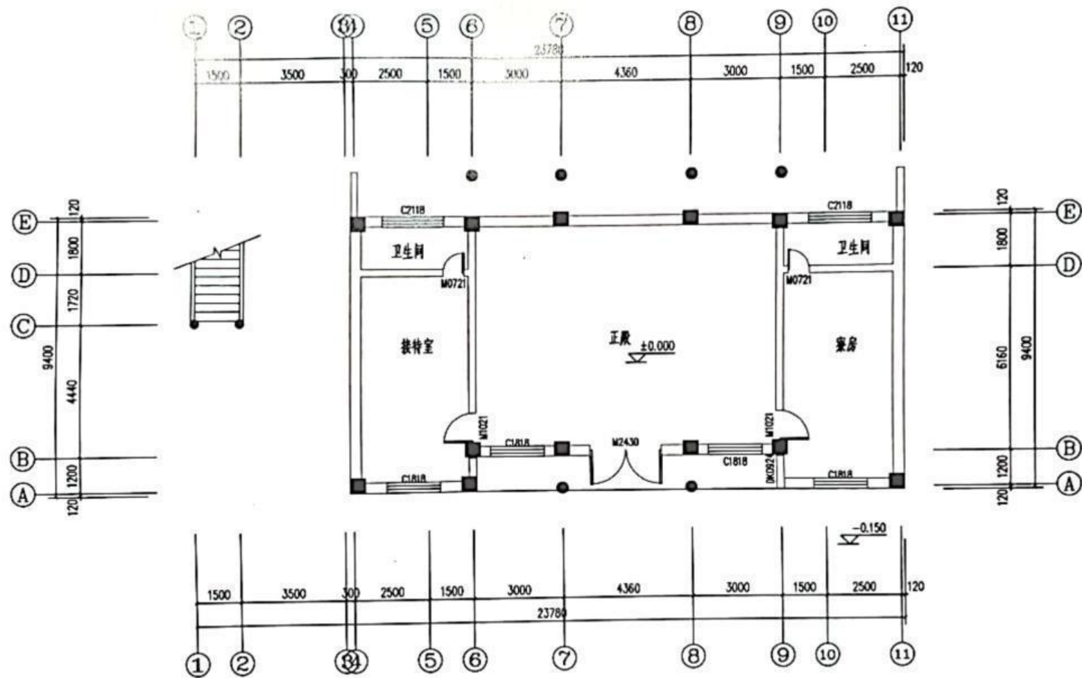
西福庵一层平面图
