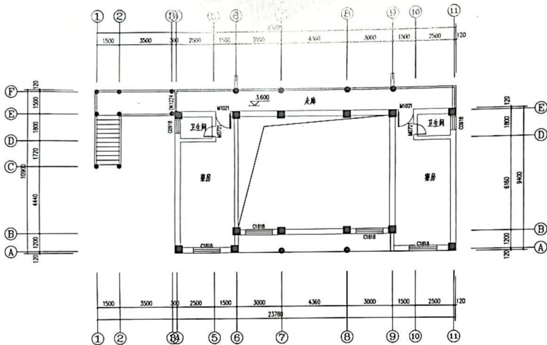
西福庵二层平面图
